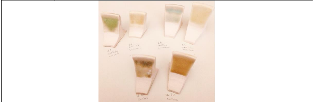
Muestrario de celadones con carburo de silicio
