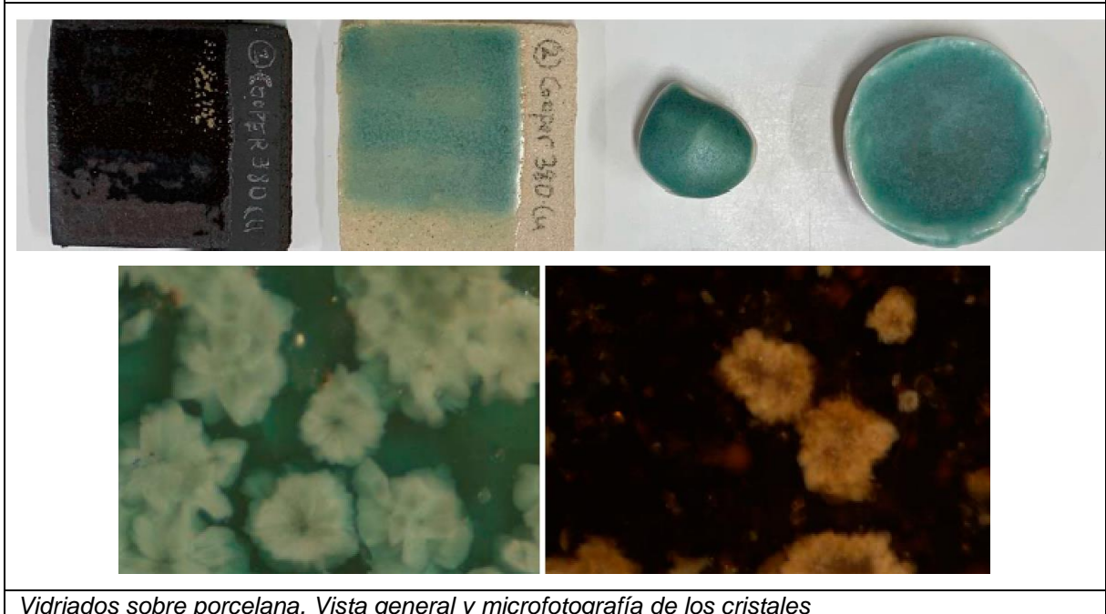
Muestrario de celadones con carburo de silicio
